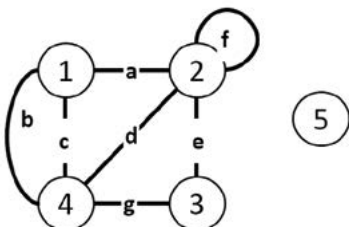
Figura 5. Grado en pseudografos no dirigidos
