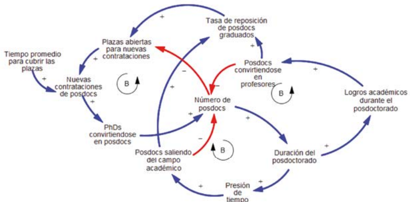
Figura 7. CLD simplificados representando los principales bucles que impactan en el crecimiento de posdocs en Estados Unidos
